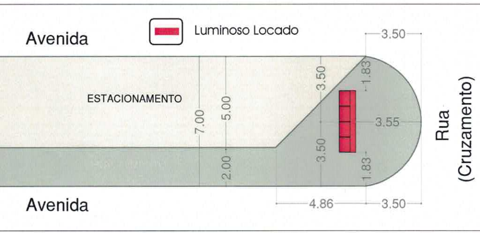
Locação dos Luminosos no Canteiro das Avenidas 1:3000
