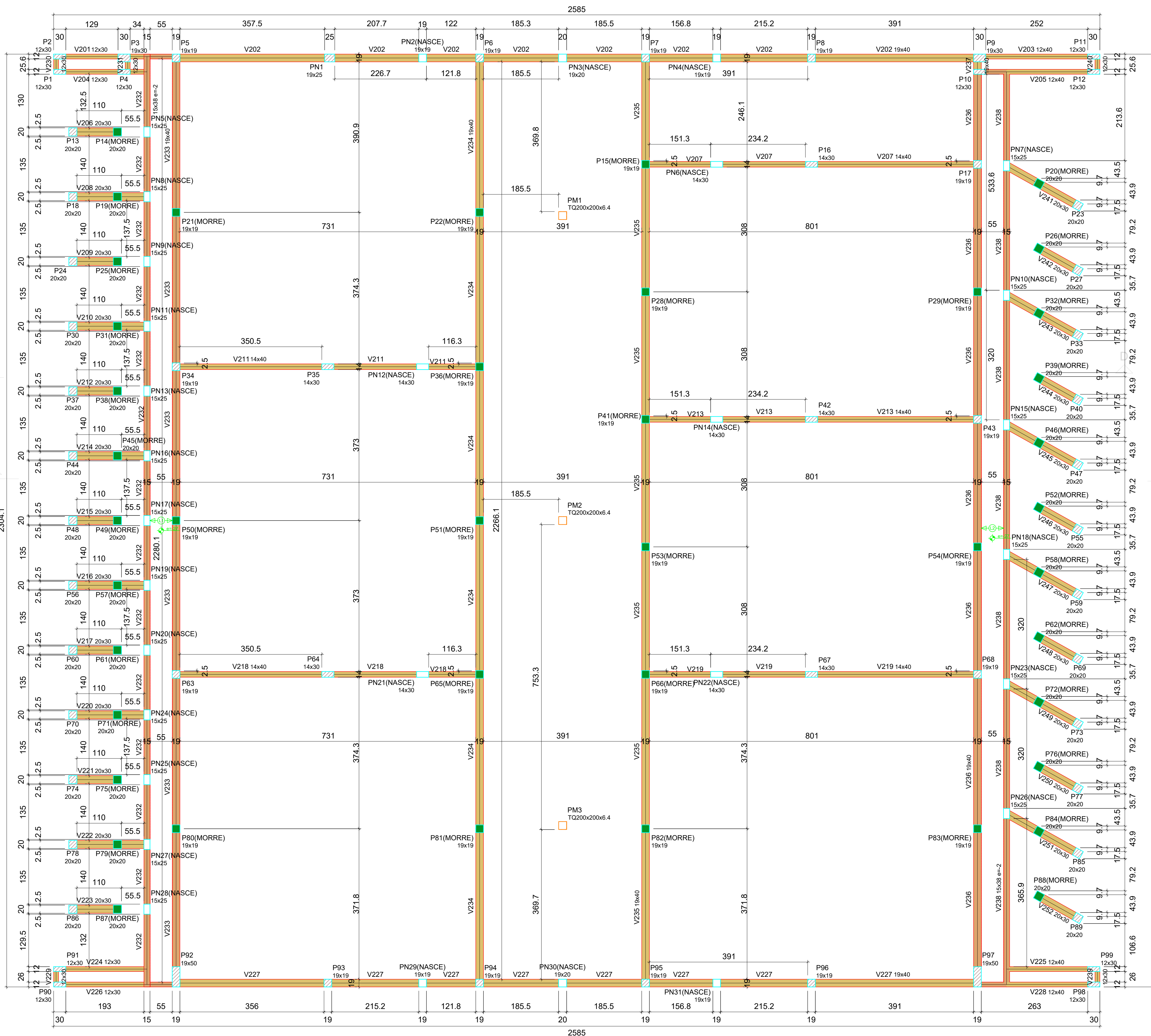
Forma do pavimento NIVEL350 (Nível 350) escala 1:50
