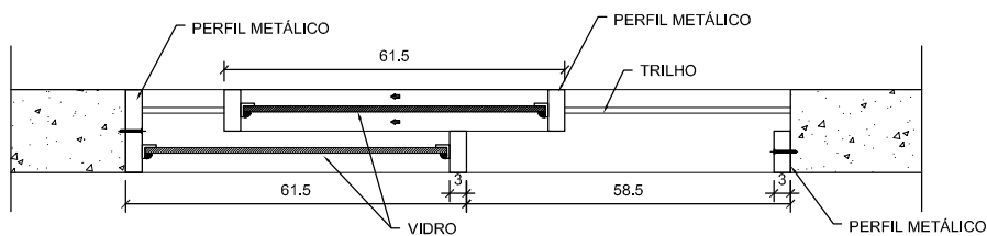
PLANTA ESC. 1/10
