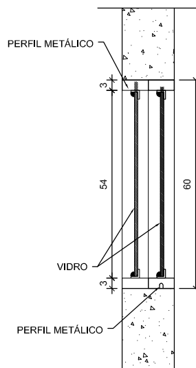
SEÇÃO 1-1 ESC. 1/10
