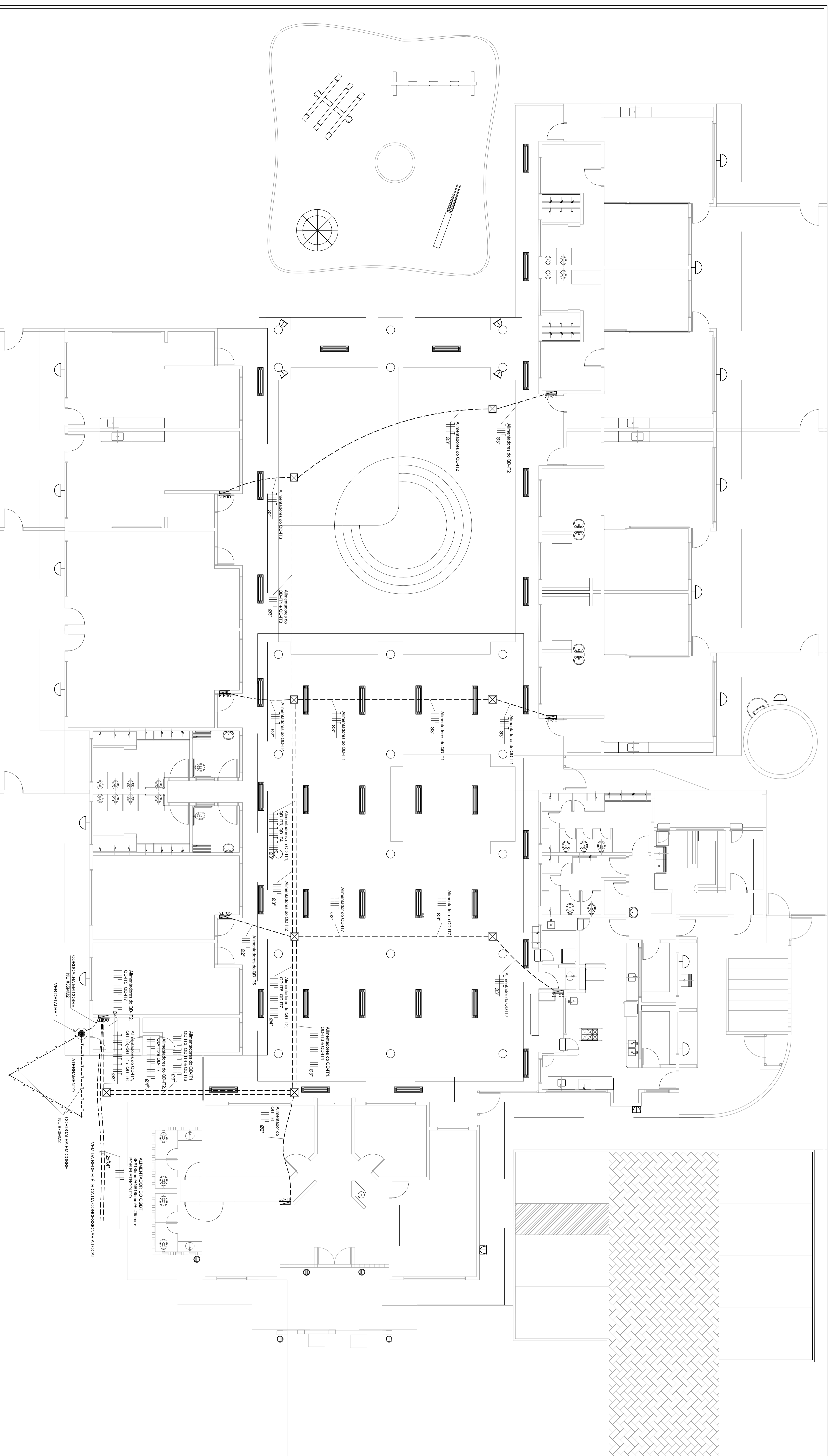
ALIMENTAÇÃO DOS QUADROS E LOCAÇÃO DAS LUMINÁRIAS EXTERNAS ESCALA: 1/75
