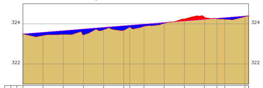
Perfil Longitudinal – RUA DILMA
