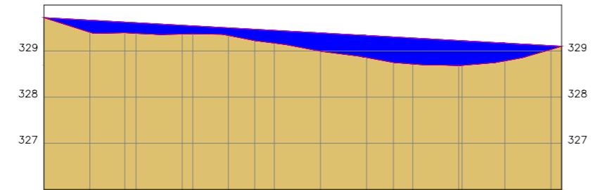
Perfil Longitudinal Lída
