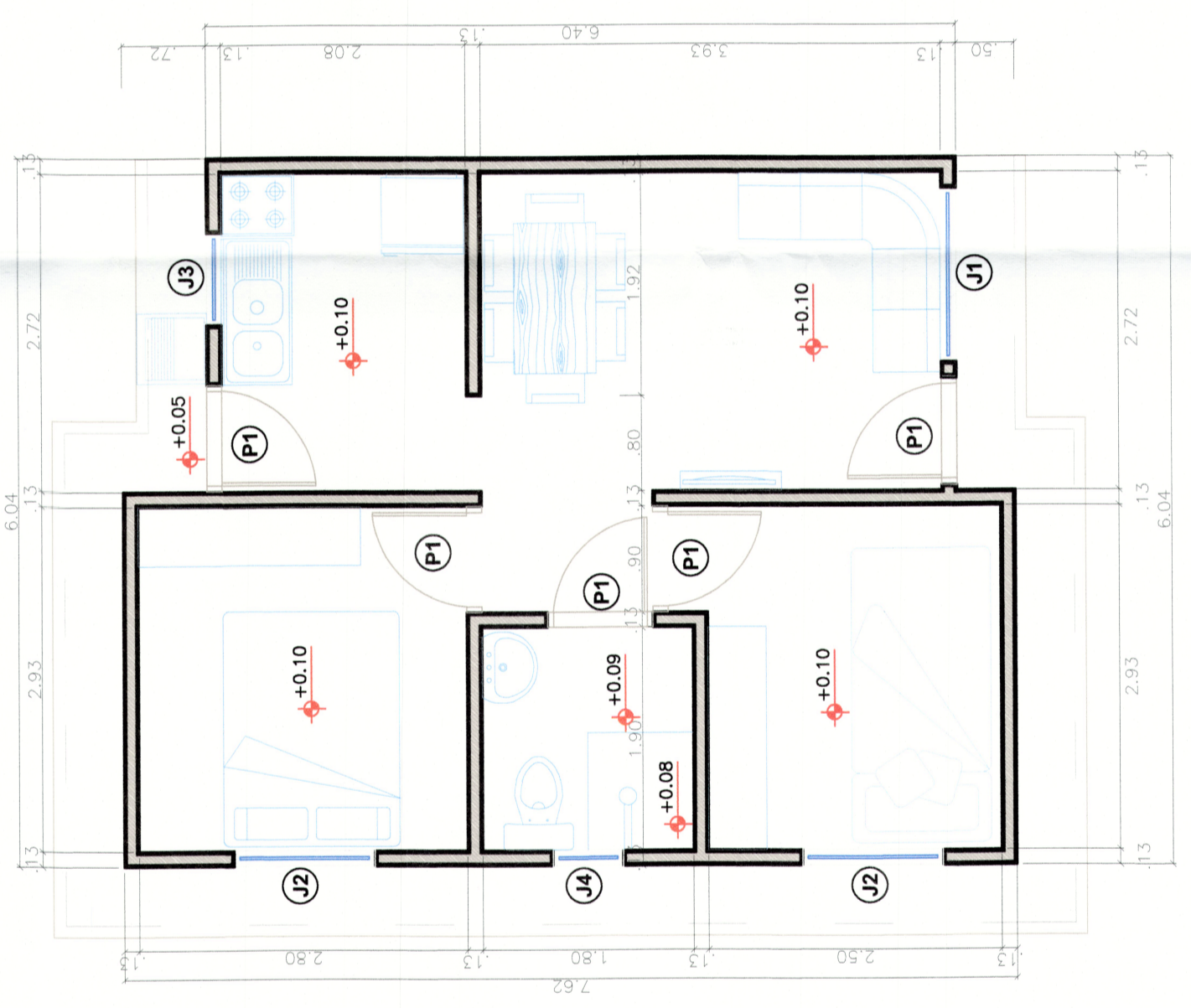
PLANTA BAIXA LOTE 010 - QUADRA 074 Esc: 1:50
