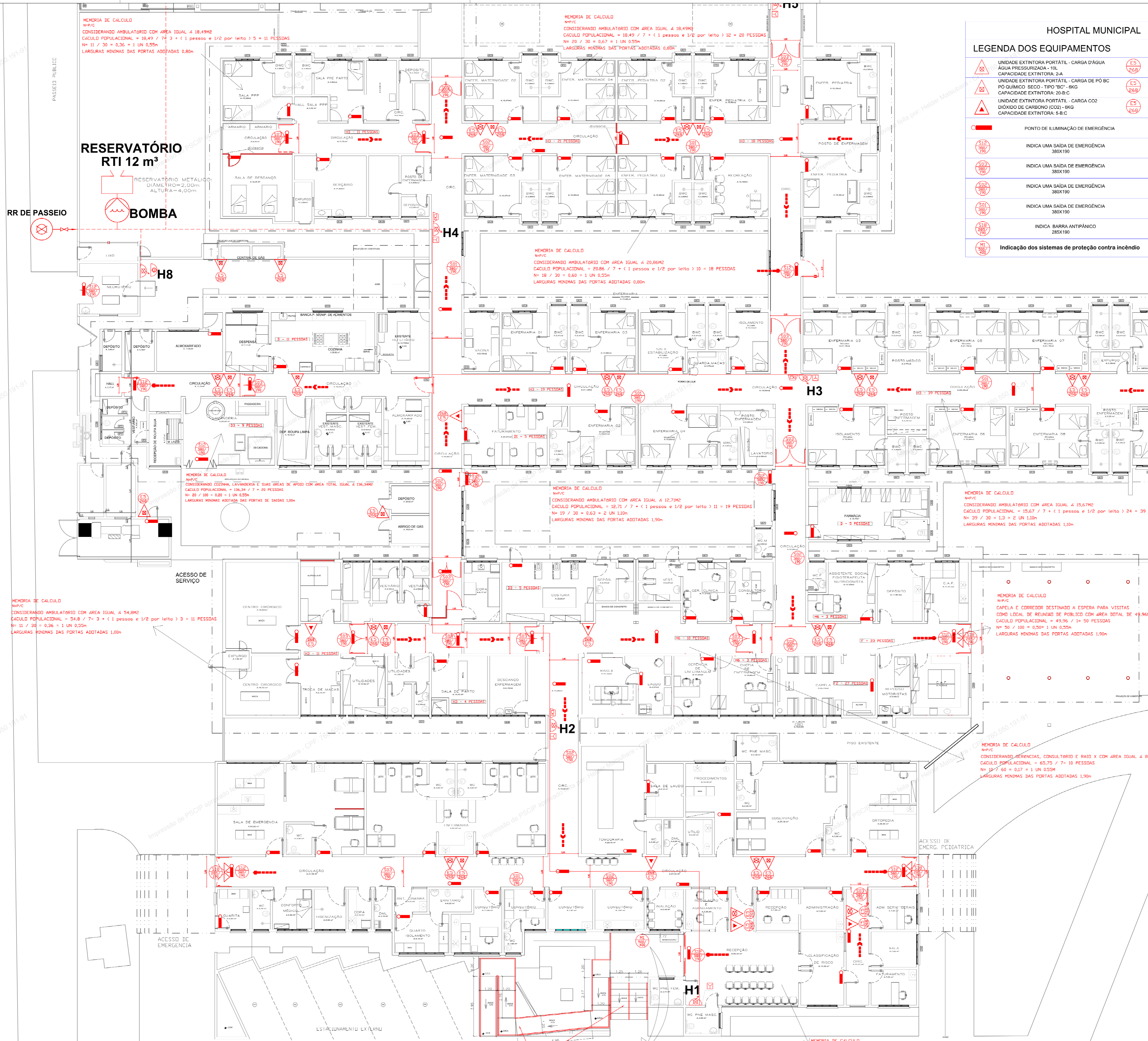
PLANTA DE PREVENTIVOS - BLOCO 01 Escala 1:125
