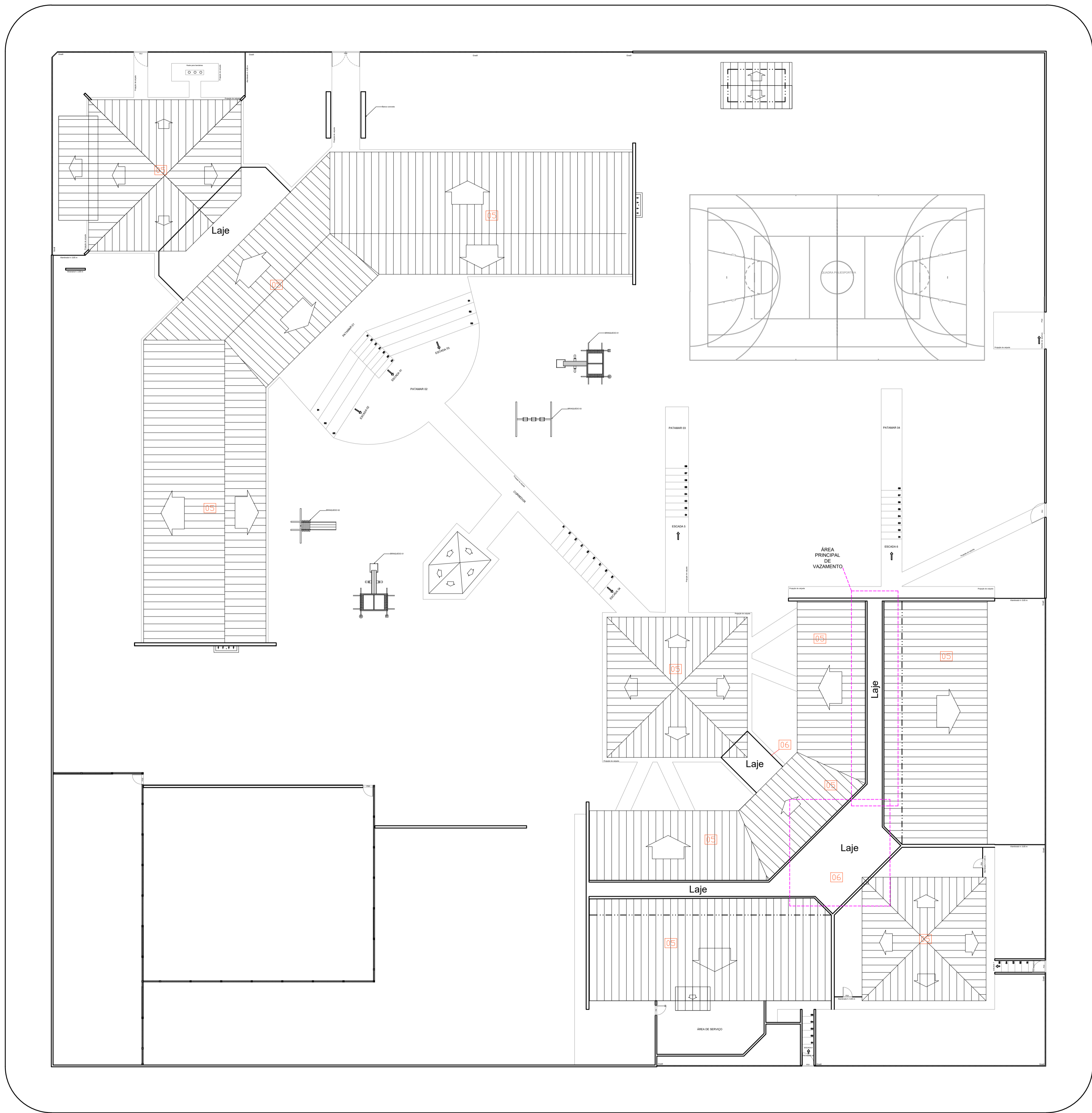
3 PLANTA DE COBERTURA REFORMA ESCALA 1:200
