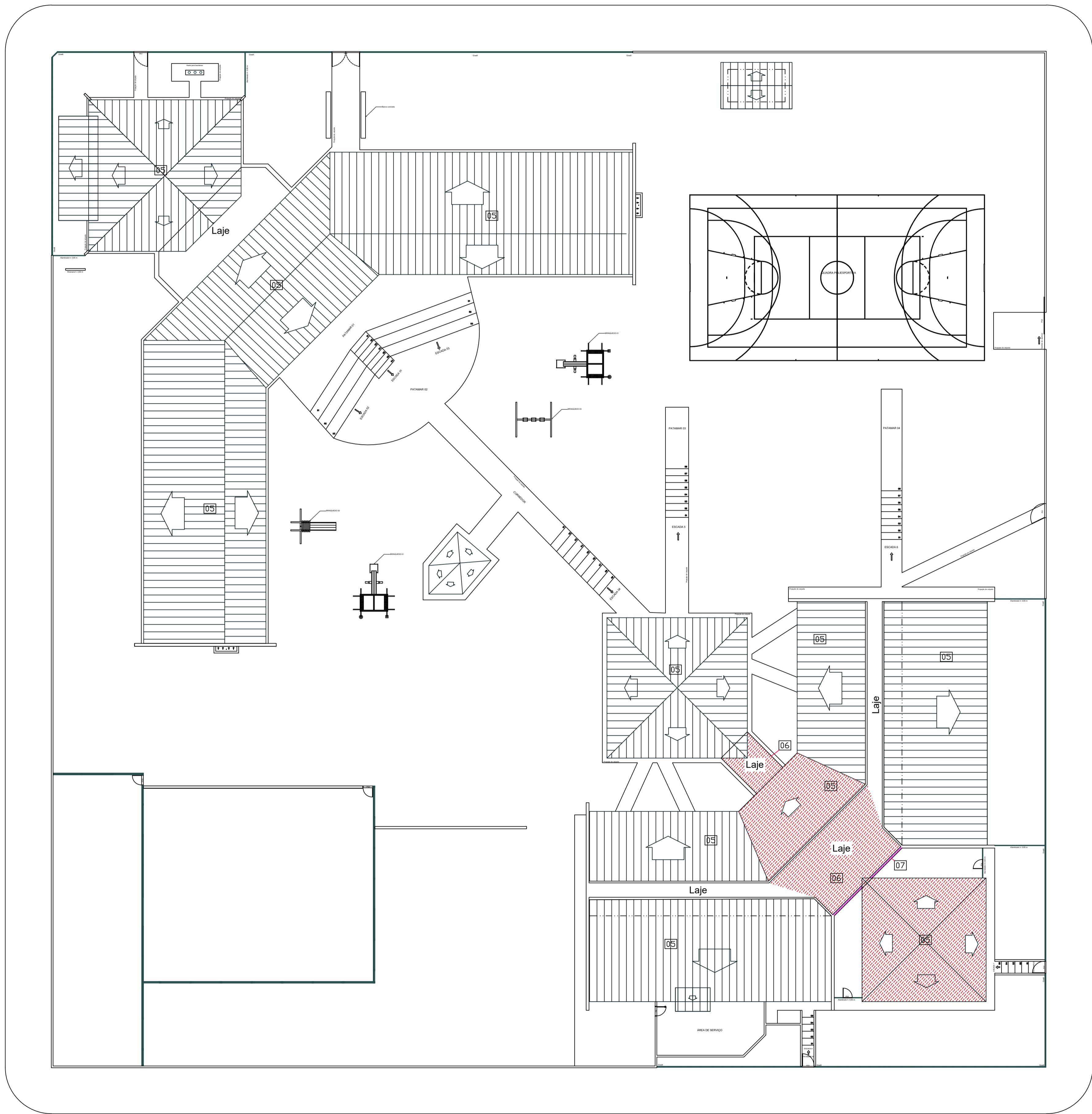
1 PLANTA DE COBERTURA REFORMA ESCALA 1:200
