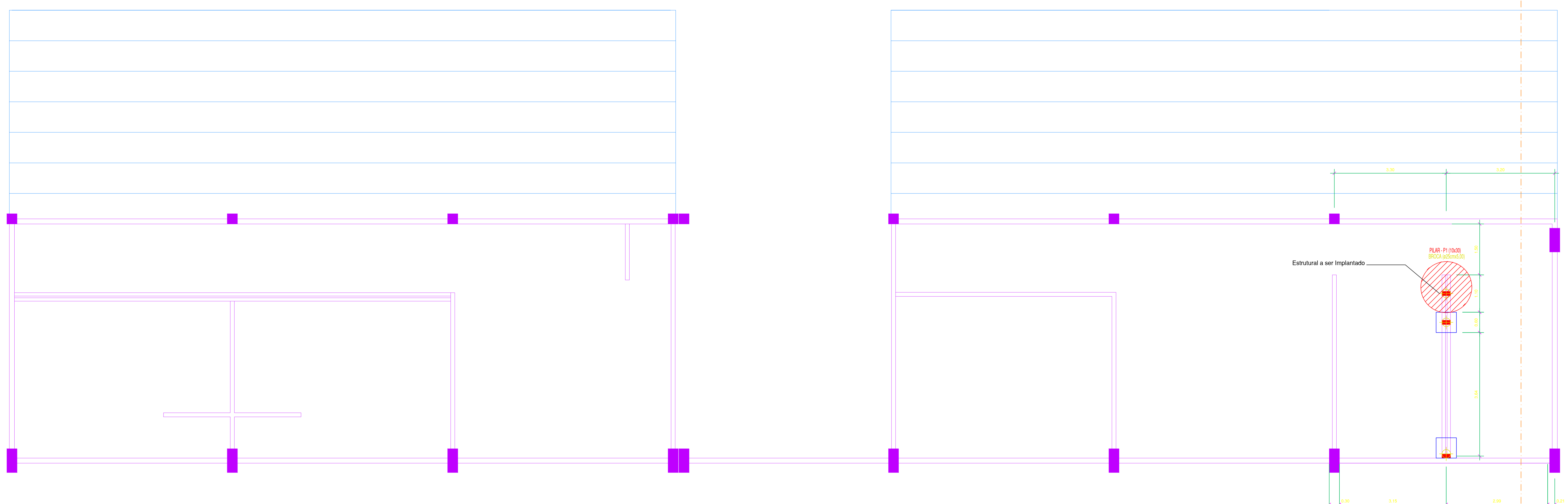
FUNDAÇÕES E VIGAS BALDRAME Escala 1/25
