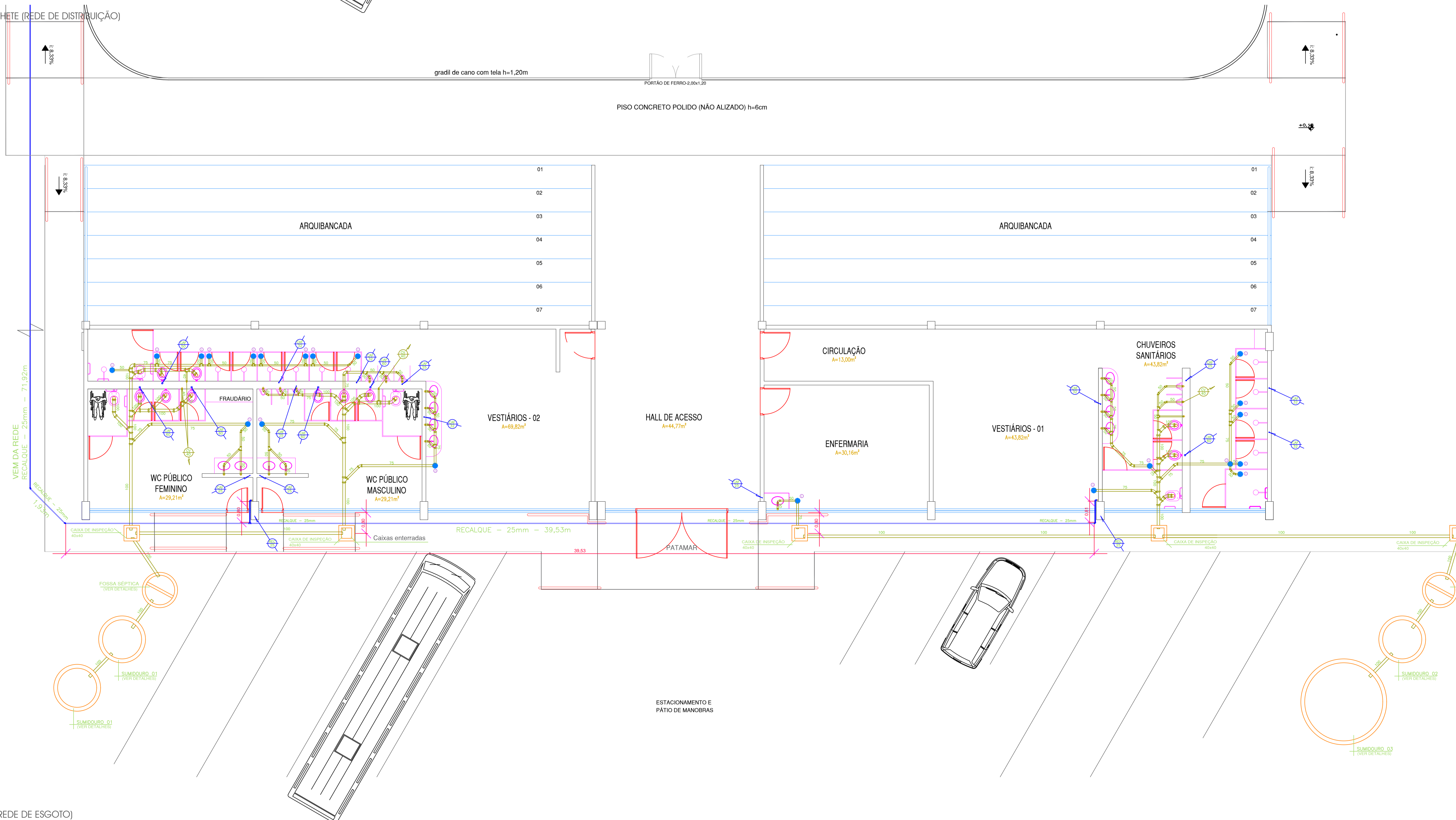
PLANTA BAIXA (REDE DE ESGOTO) Escala 1:75
