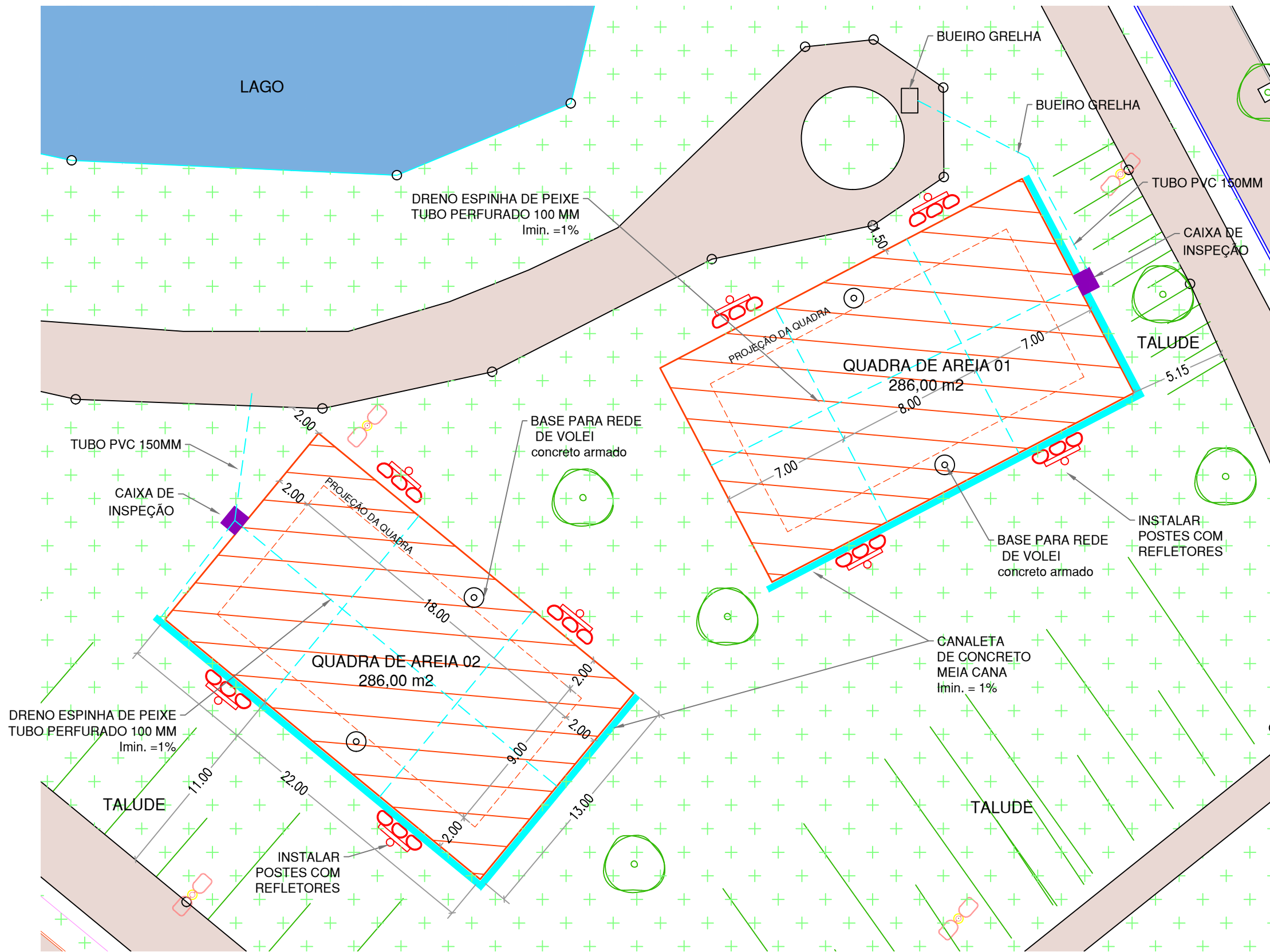
IMPLANTAÇÃO QUADRA DE AREIA escala 1:250
