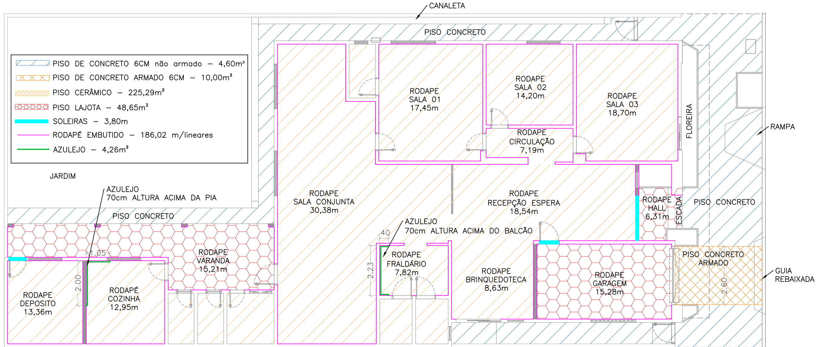
PLANTA esc 1:150
