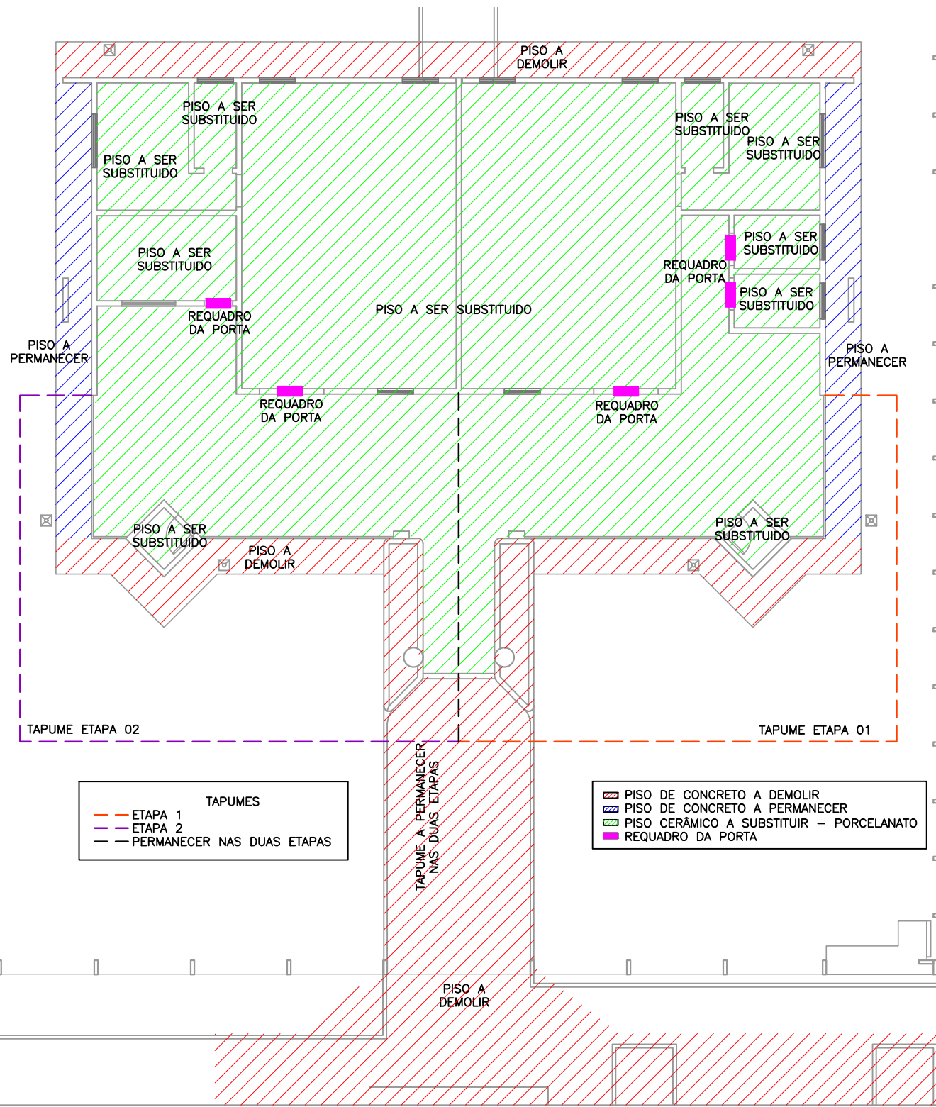
PISOS E TAPUMES esc 1:150
