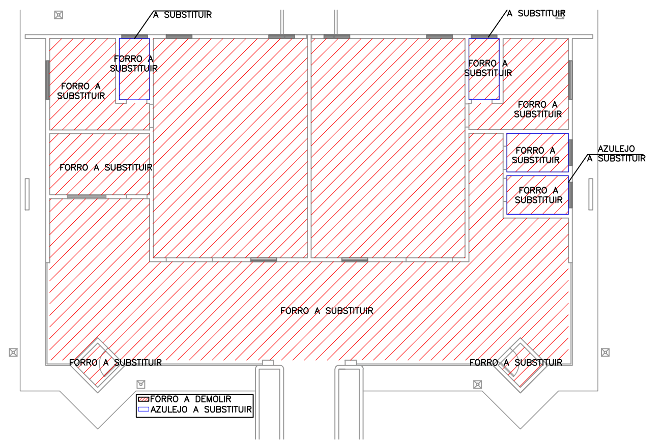
SUBSTITUIÇÃO DO FORRO PVC SUBSTITUIÇÃO DO AZULEJO - REVESTIMENTO DE PORCELANATO EM PAREDE esc 1:150
