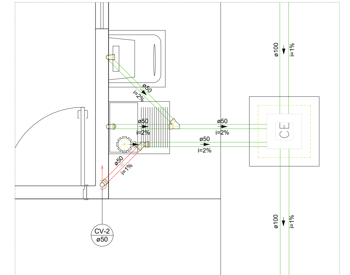
Detalhe SAN-2 Escala 1:25
