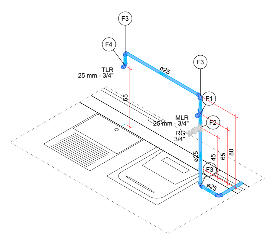
Detalhe HID-2 Escala 1:25
