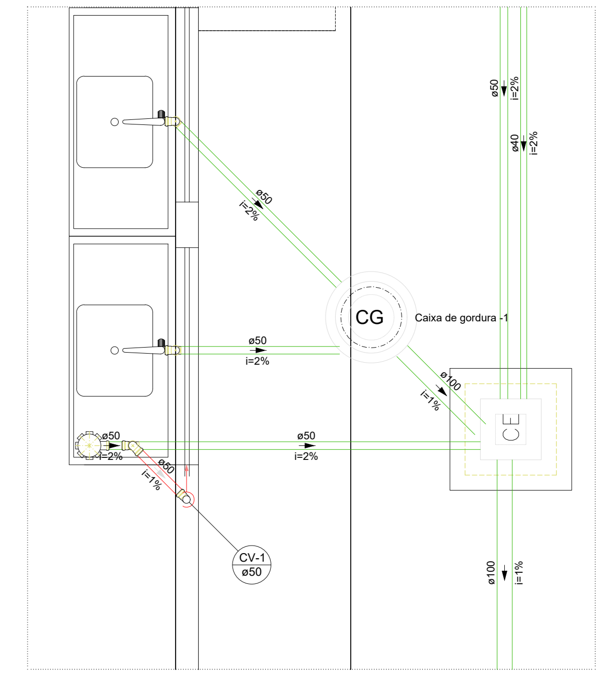
Detalhe SAN-1 Escala 1:25
