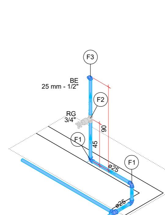
Detalhe HID-3 Escala 1:25
