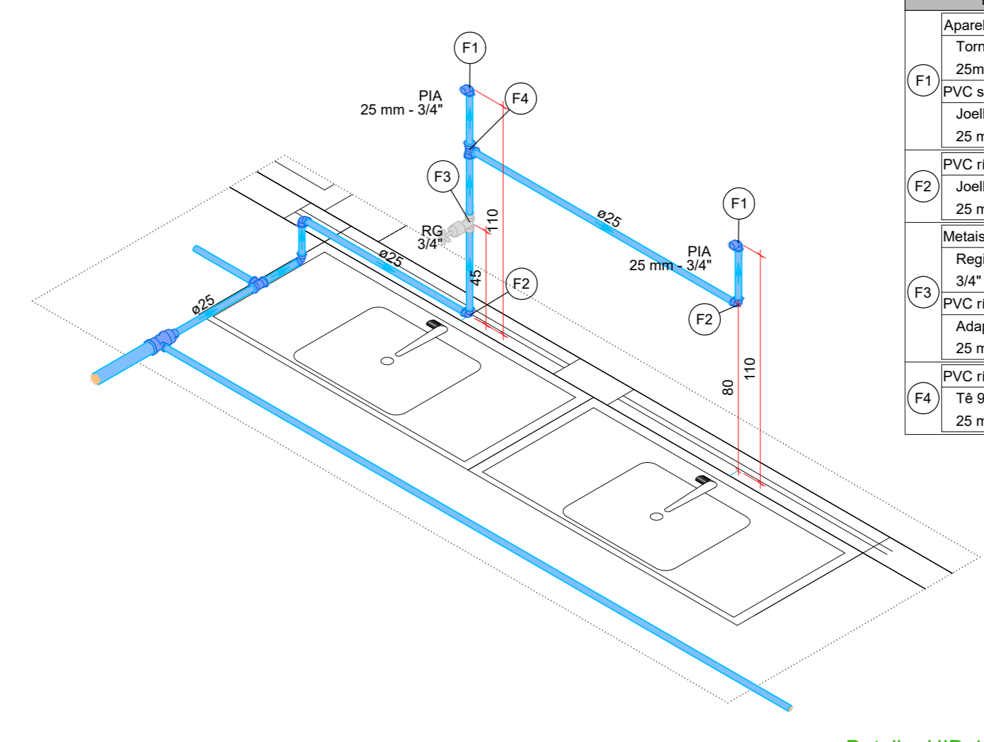
Detalhe HID-1 Escala 1:25
