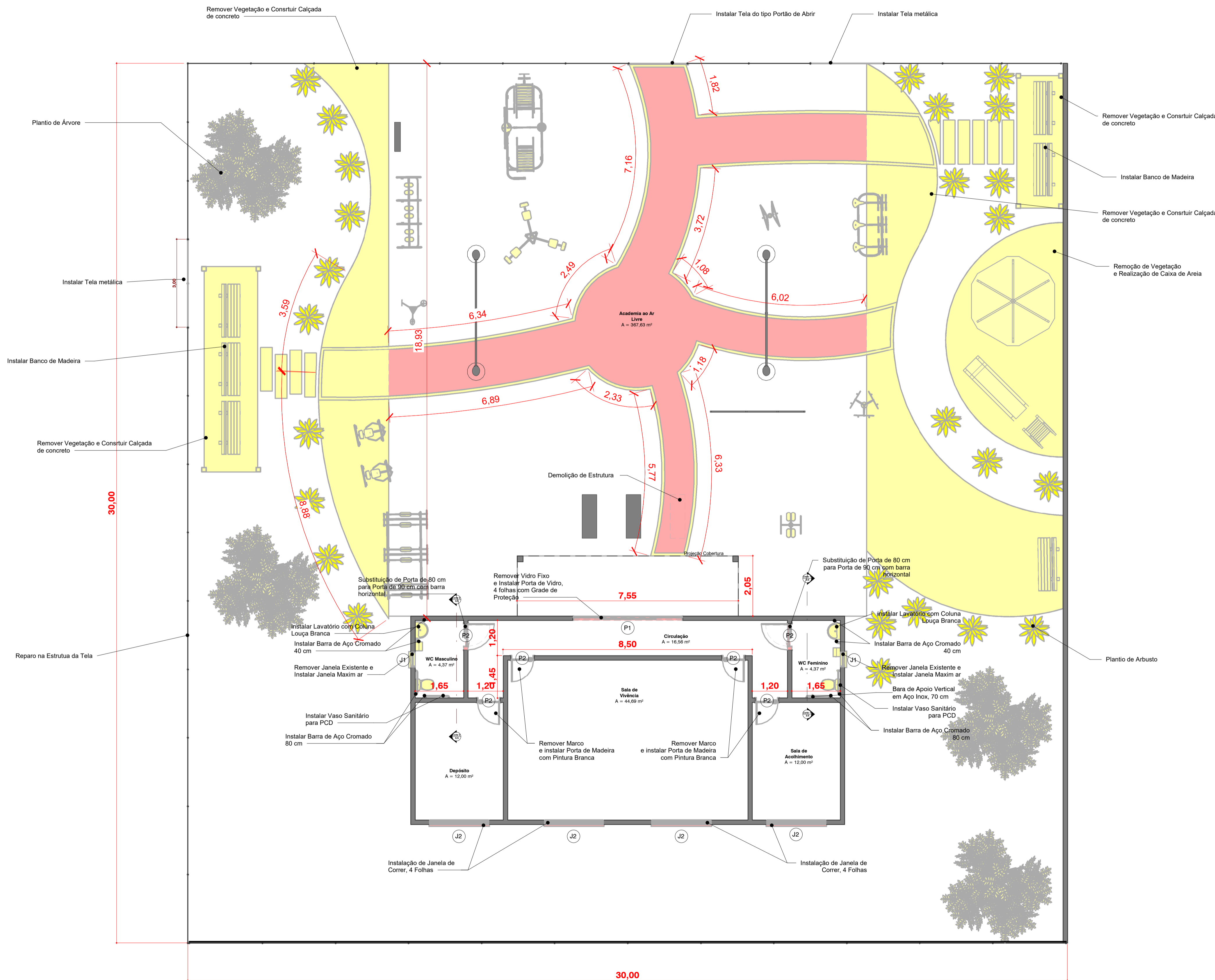
1 Planta Baixa Construir/Demolir 1 : 75
