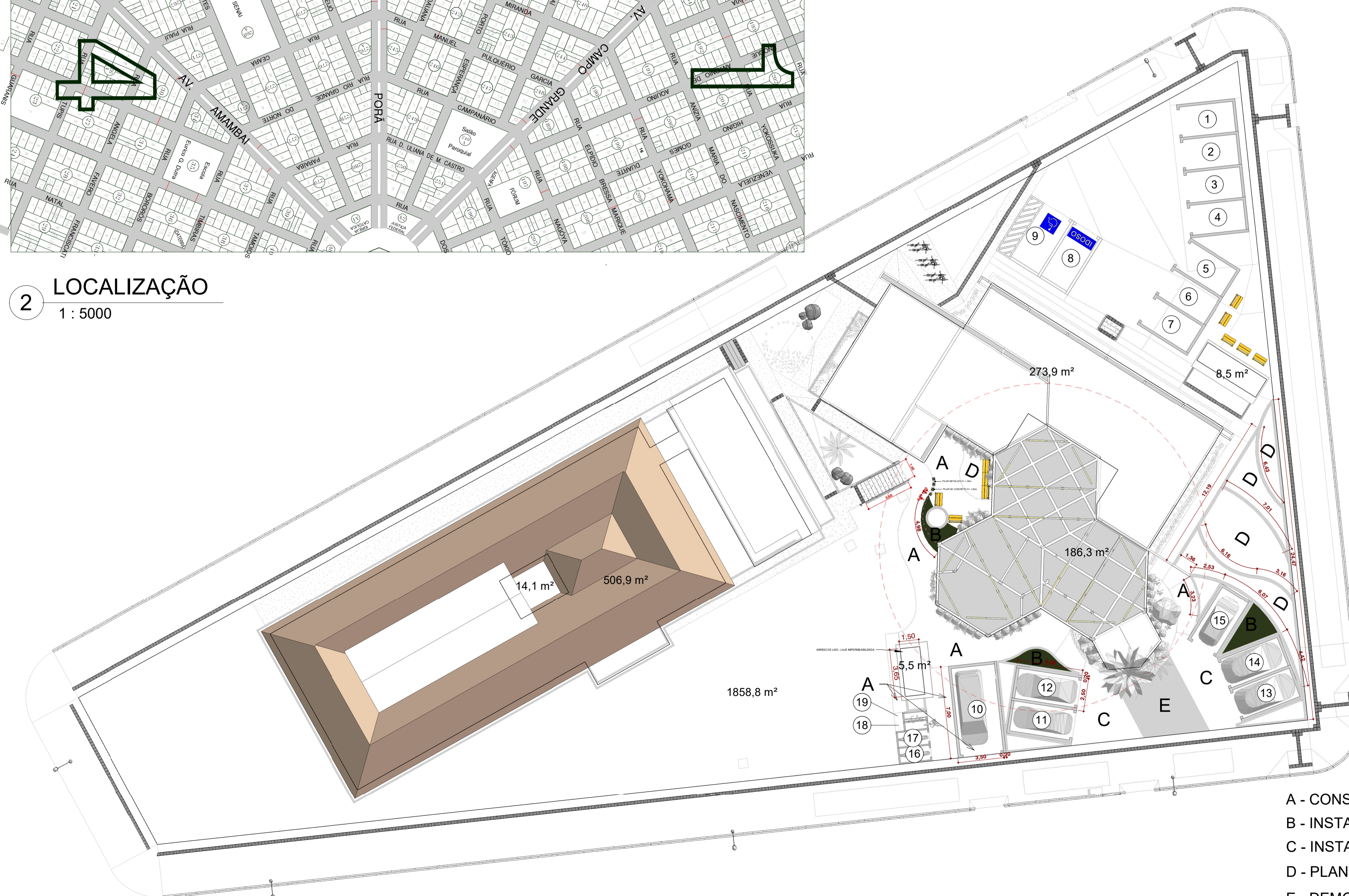
1 IMPLANTAÇÃO 1 : 200
