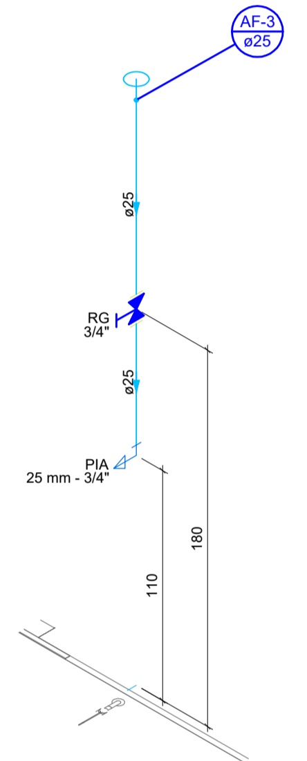
ARMAZENAGEM Detalhe HID-4 Escala 1:25
