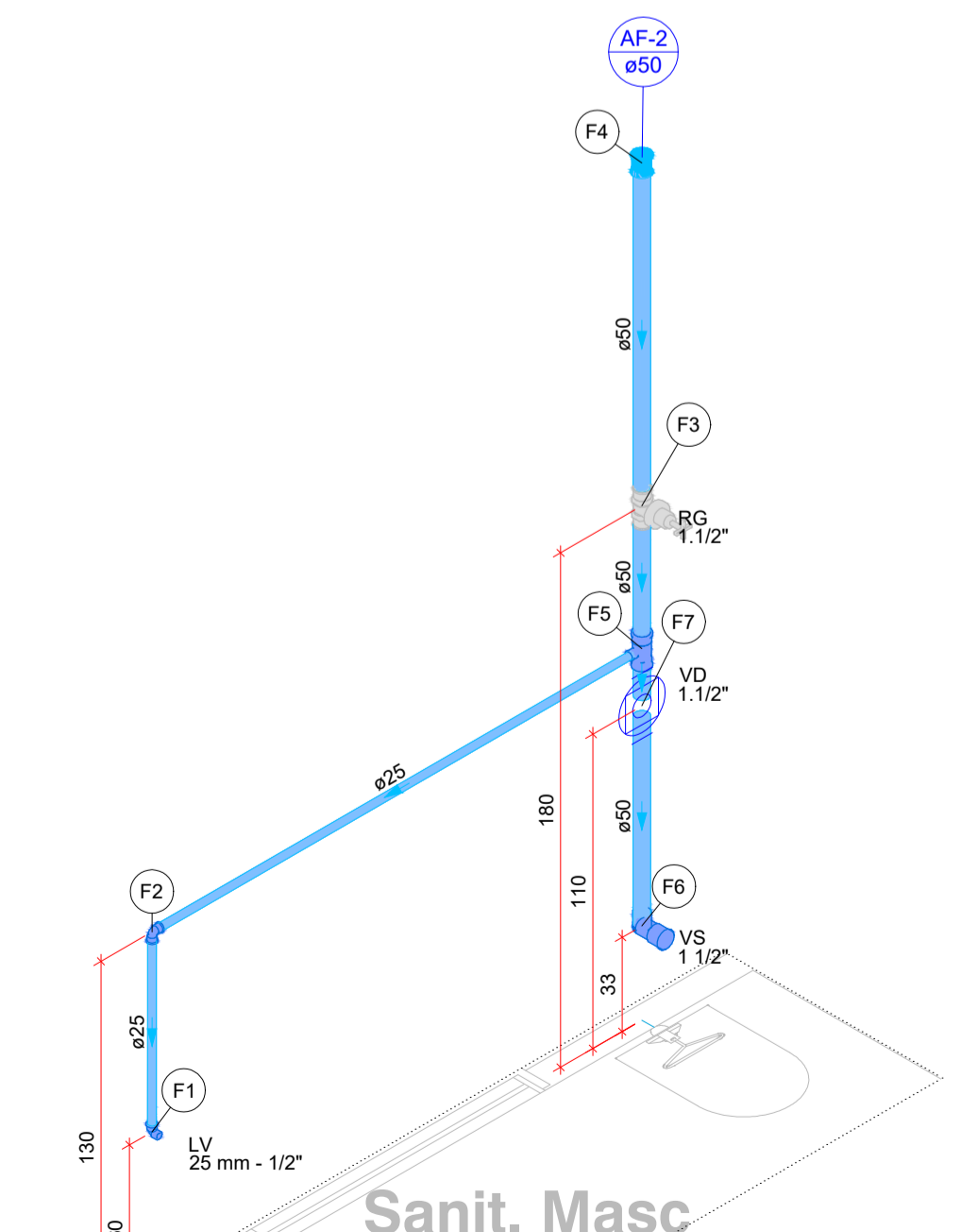
Detalhe HID-2 Escala 1:25
