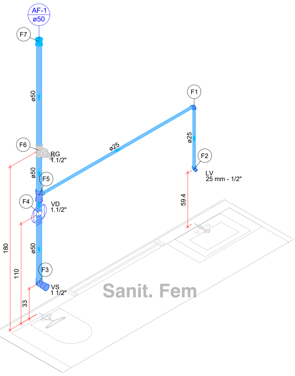
Detalhe HID-1 Escala 1:25
